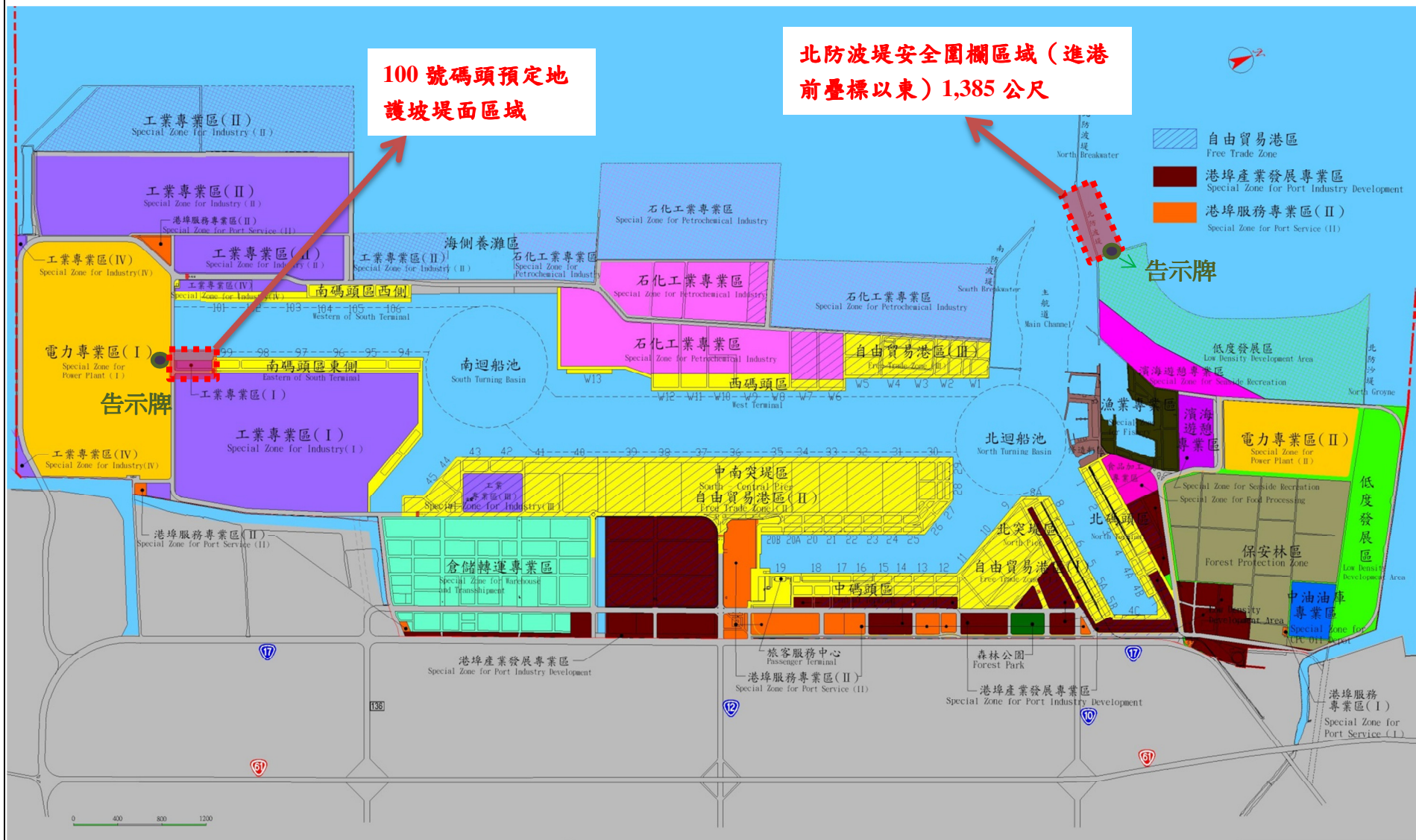
臺中港整體規劃平面配置圖 Taichung Harbor Master Plan
